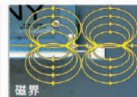
磁界
